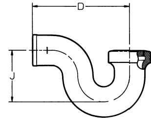
TAP P-TRAP
