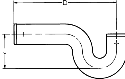
LONG P-TRAP
