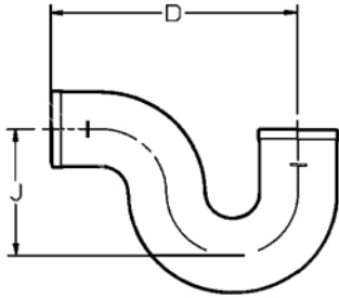
P-TRAP
