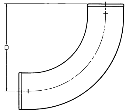
LONG SWEEP
