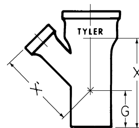
TAPPED WYE
