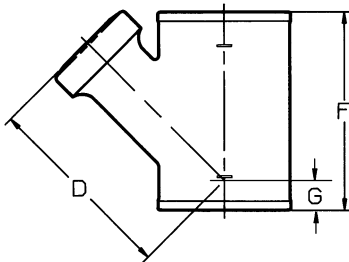
TAP WYE
