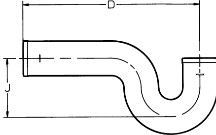
LONG P-TRAP
