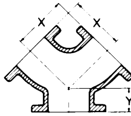
True Wye
